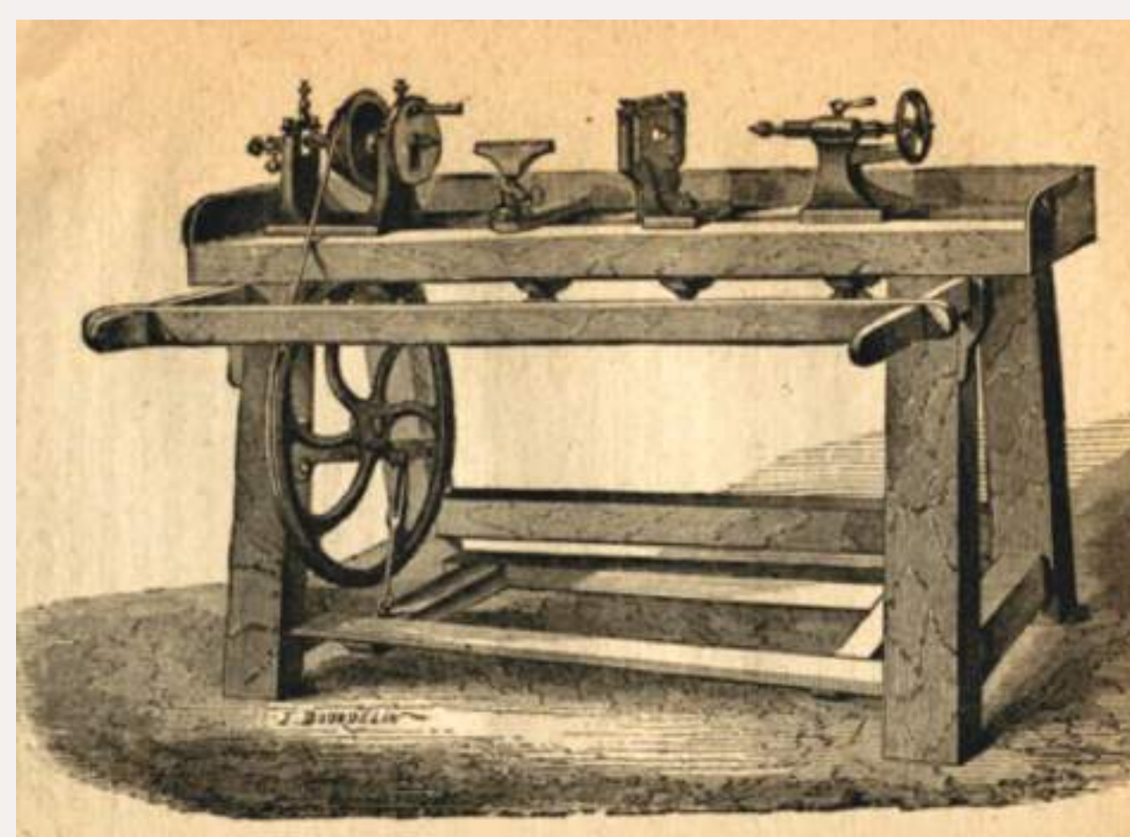
Antiguas herramientas de cerrajería y forja, según el Manual del Herrero y Cerrajero de Marcelino García López, de 1880 (BNE). De izquierda a derecha y de arriba a abajo: torno, yunque, tenazas, máquina de cepillar o tornillo limador, tornillo, máquina para cortar y taladrar chapas, berbiquí.
